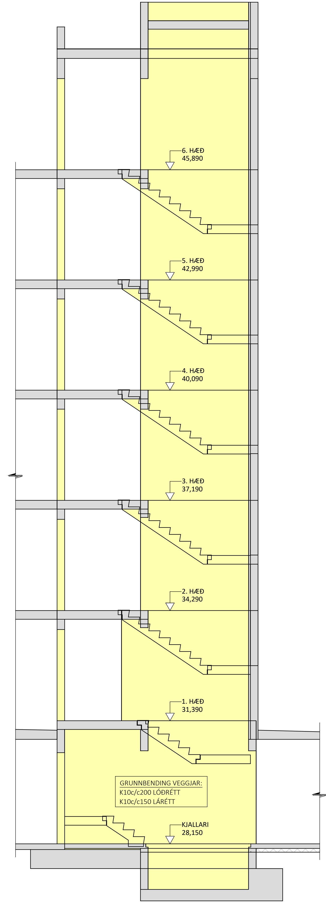
HLIÐARMYND VEGGIAR V107 & V307 - M1:50: PYKKT VEGGIAR: 200mm
