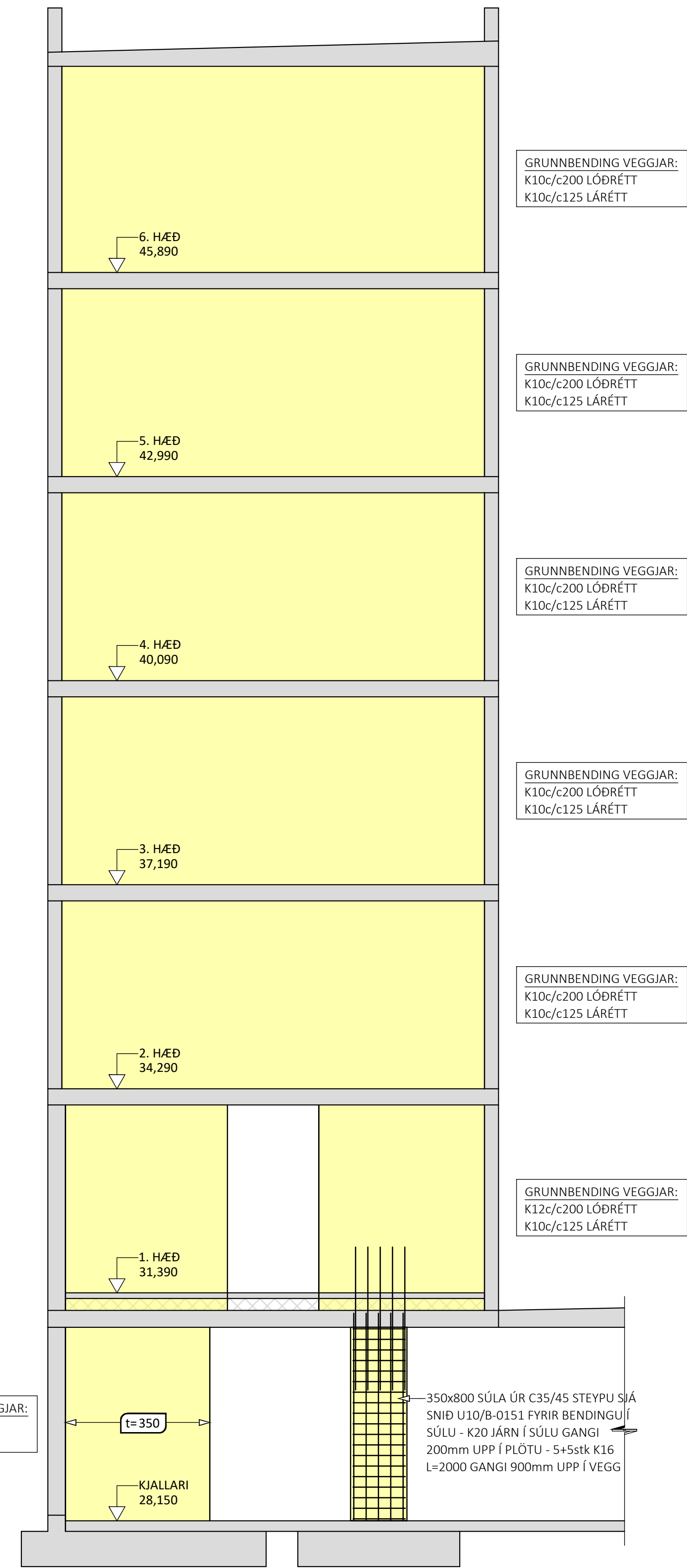
HLIÐARMYND VEGGIAR V106 & V306 - M1:50: PYKKT VEGGIAR: 200mm NEMA ANNAD SÉ SÉRSTAKLEGA TEKID FRAM
