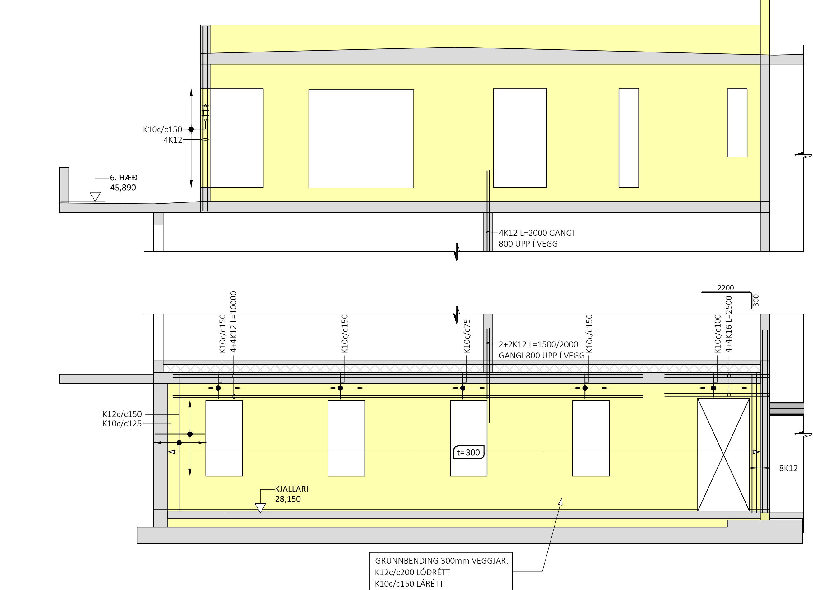
HLIÐARMYND VEGGJAR V007 - M1:50: PYKKT VEGGJAR: 200mm NEMA ANNAD SÉ SÉRSTAKLEGA TEKID FRAM
