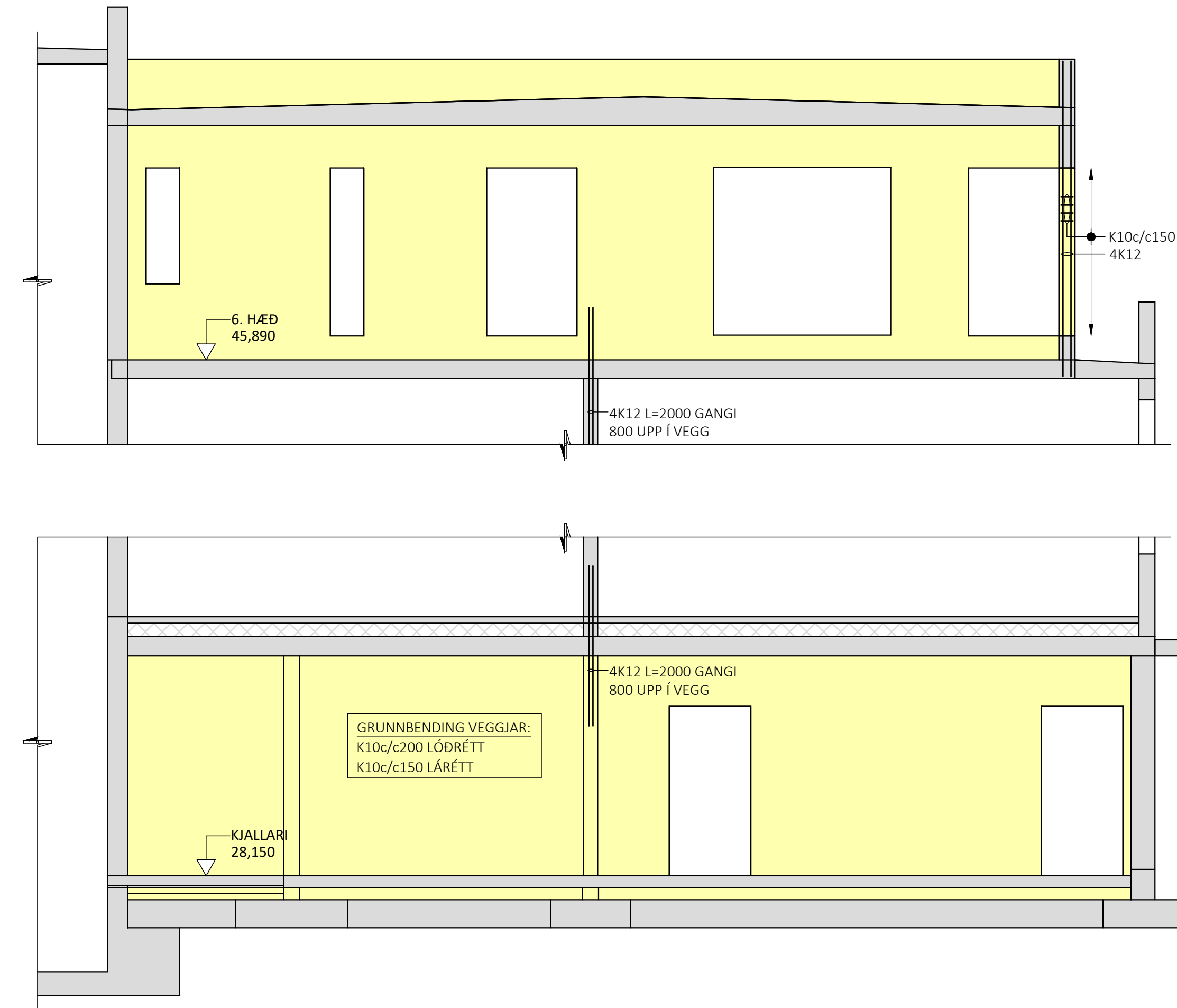
HLIÐARMYND VEGGJAR V208 - M1:50: PYKKT VEGGJAR: 200mm
