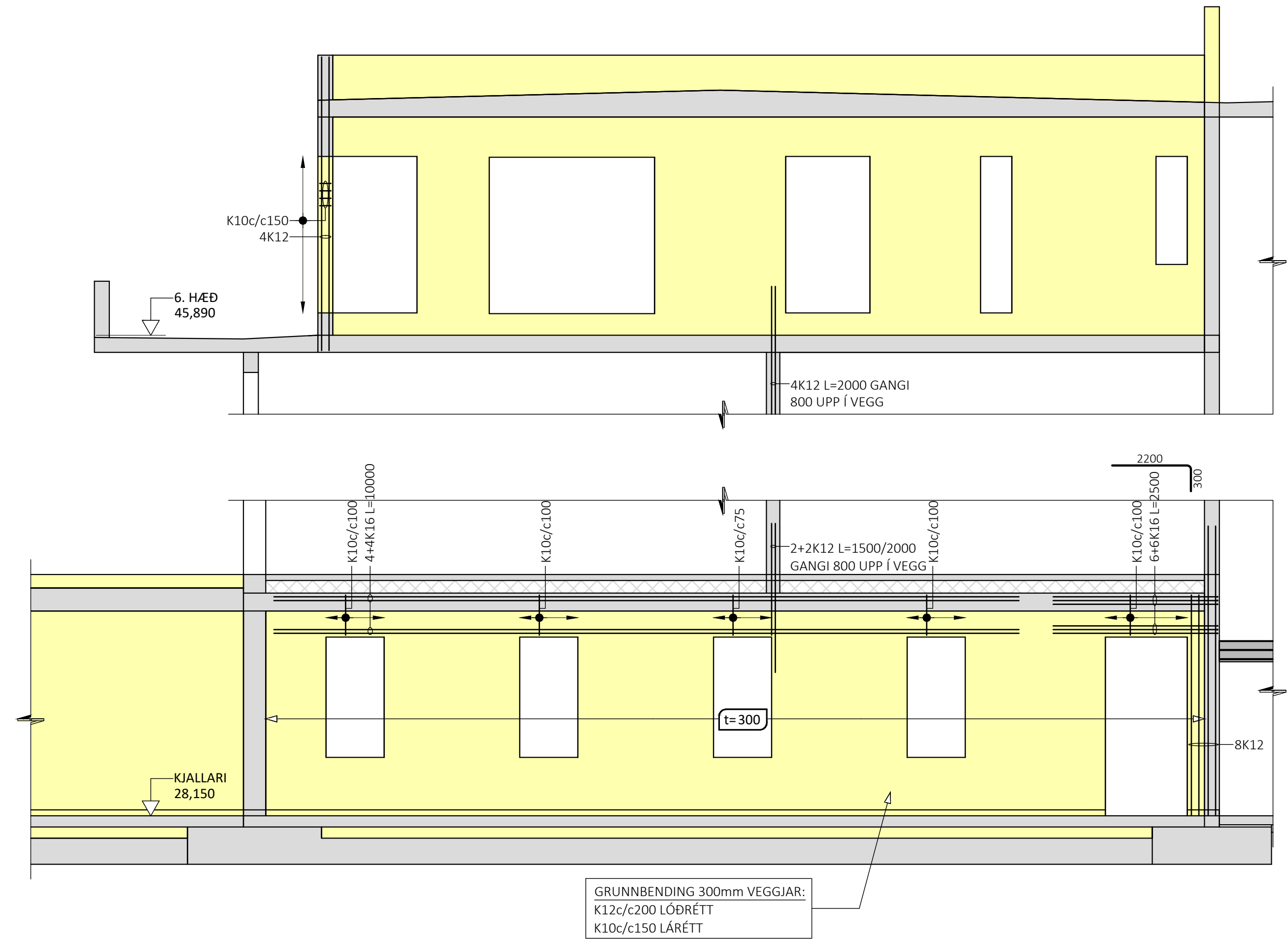
HLIÐARMYND VEGGJAR V207 - M1:50: PYKKT VEGGJAR: 200mm NEMA ANNAD SÉ SÉRSTAKLEGA TEKID FRAM
