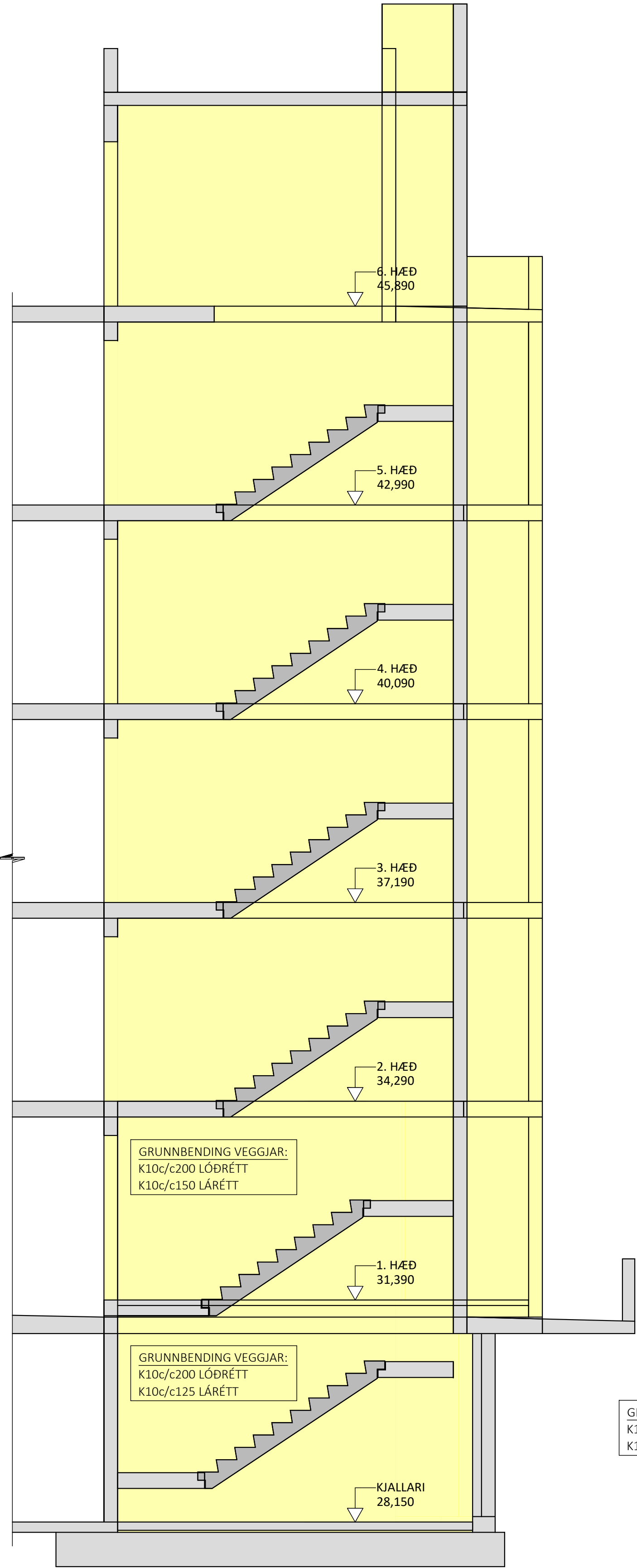
HLIÐARMYND VEGGIAR V105 & V305 - M1:50: PYKKT VEGGIAR: 200mm
